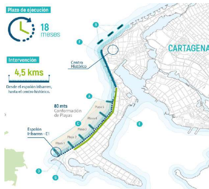
FIGURA 1. Alcance de obras proyectadas proyecto Protección Costera, fase 1, componente 1 (Fuente: UNGRD).
